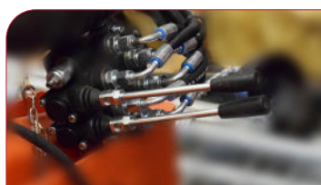
Detalle del distribuidor hidráulico.
