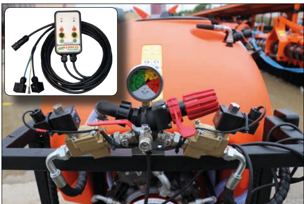
MODELOS (EL) ELECTROVÁLVULAS Y MANDOS DE CONTROL.
