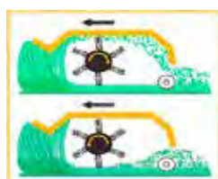
Rotación Hidráulica con dispositivo de seguridad.
